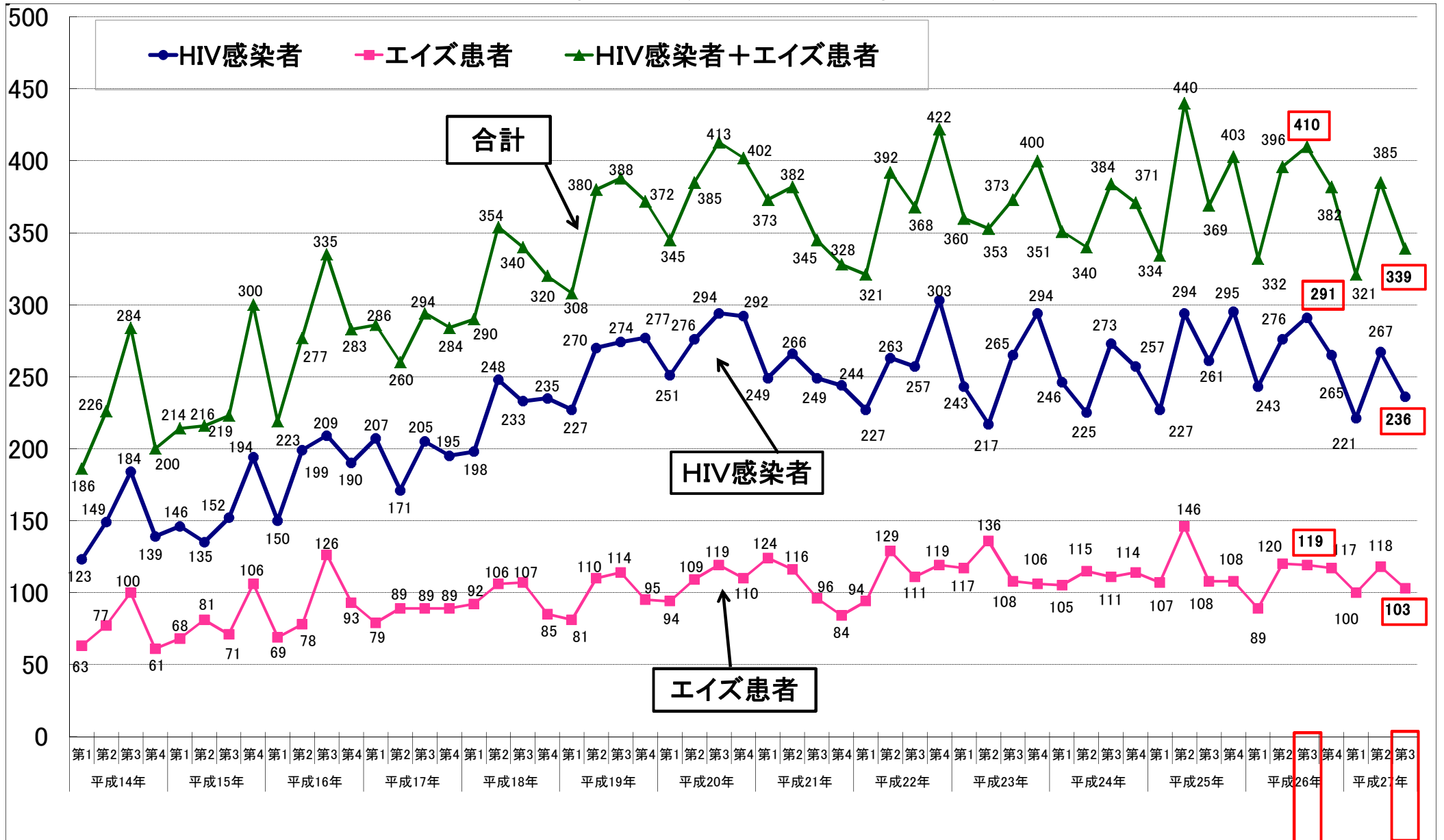
HIV感染者・エイズ患者報告件数の推移 (平成14年第1四半期～平成27年第3四半期)
